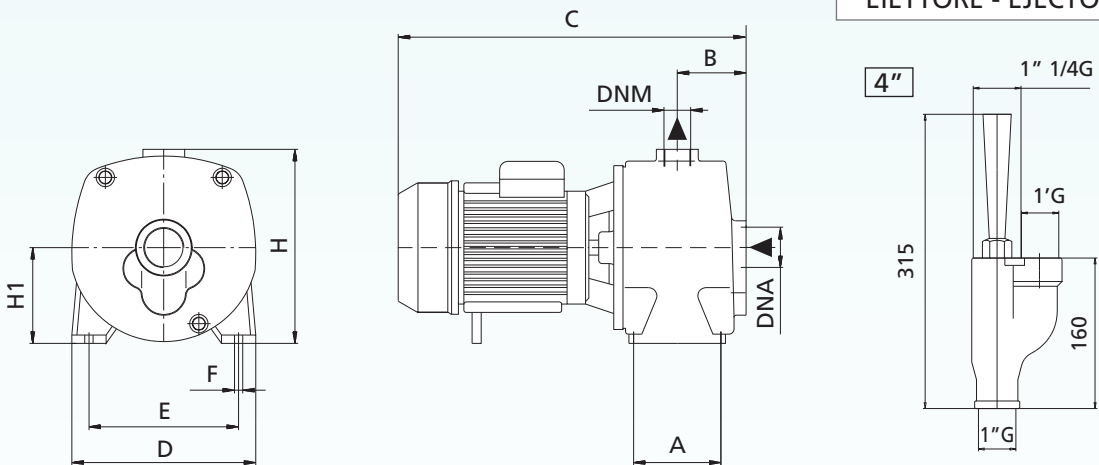
EIETTORE - EJECTOR
